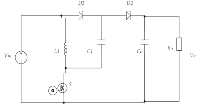
Fig 2. Luo Converter
